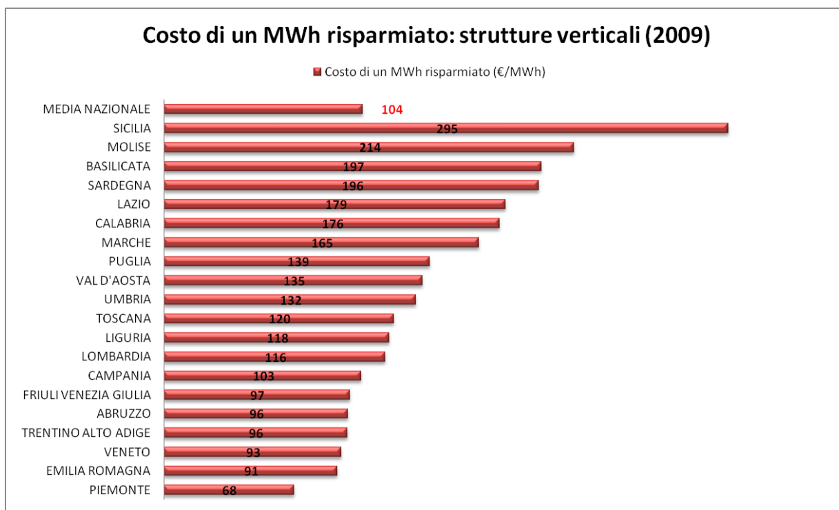
Figura 3.11 Distribuzione regionale del costo medio annuo di ogni MWh risparmiato con gli interventi
