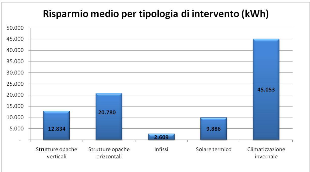
Figura 10: Risparmio medio annuo ottenuto per tipologia di intervento – Bolzano
