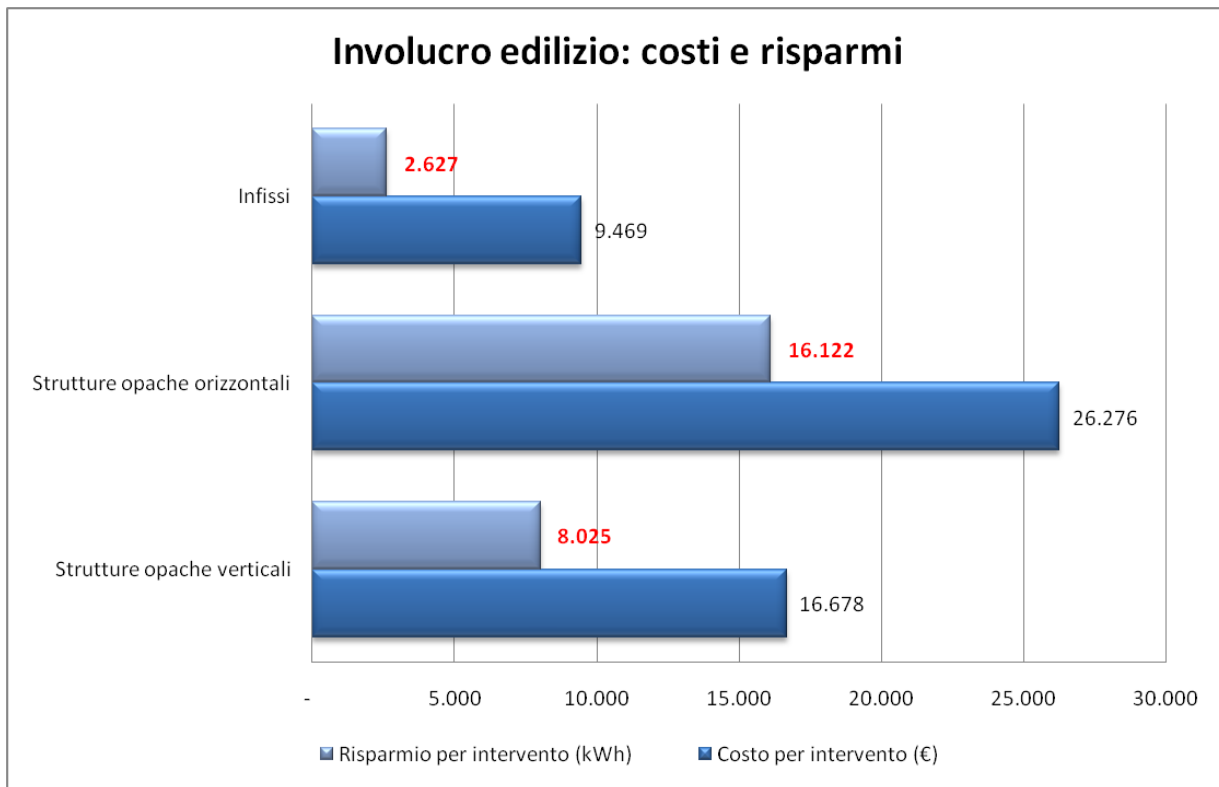
Figura 3.21 Risparmio medio per tipologia di intervento.
