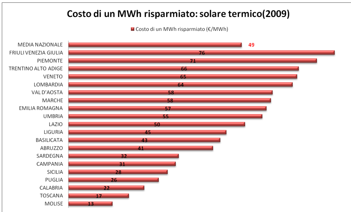
Figura 3.26 Costo medio dell'energia risparmiata con l'installazione del solare termico.
