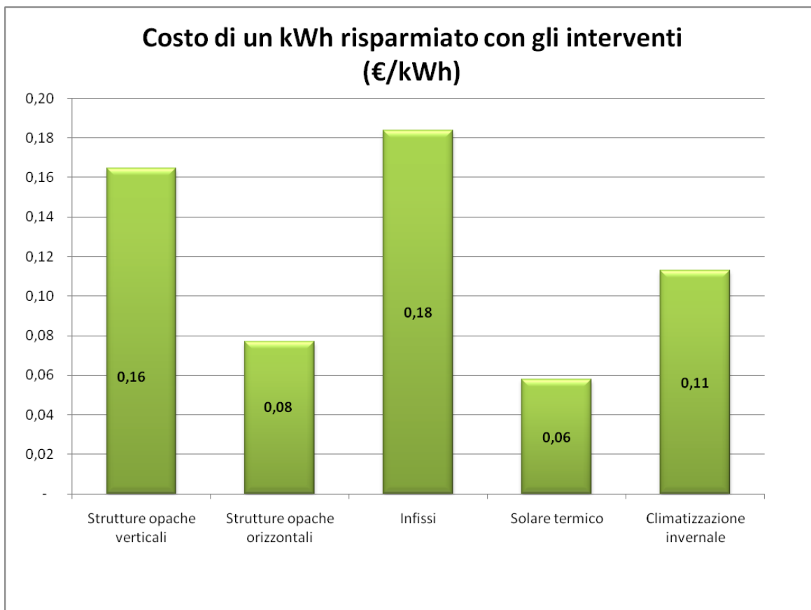
Figura 11: Costo di un MWh annuo risparmiato per tipologia di intervento – Marche
