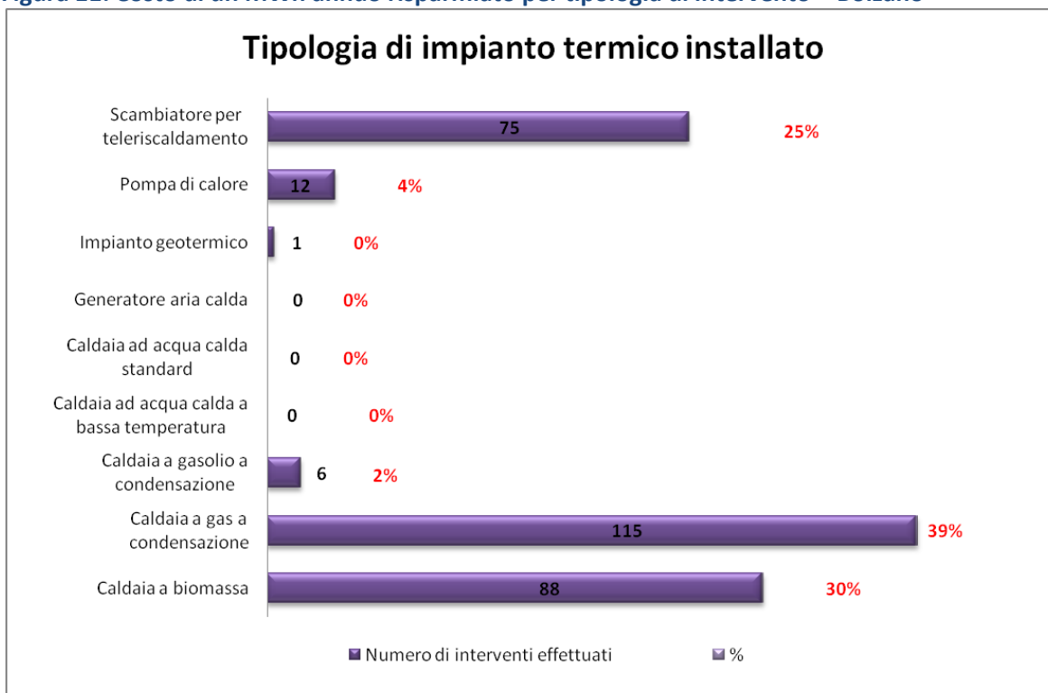
Figura 12: Distribuzione delle pratiche pervenute per tipologia di impianto termico sostituito – Bolzano
