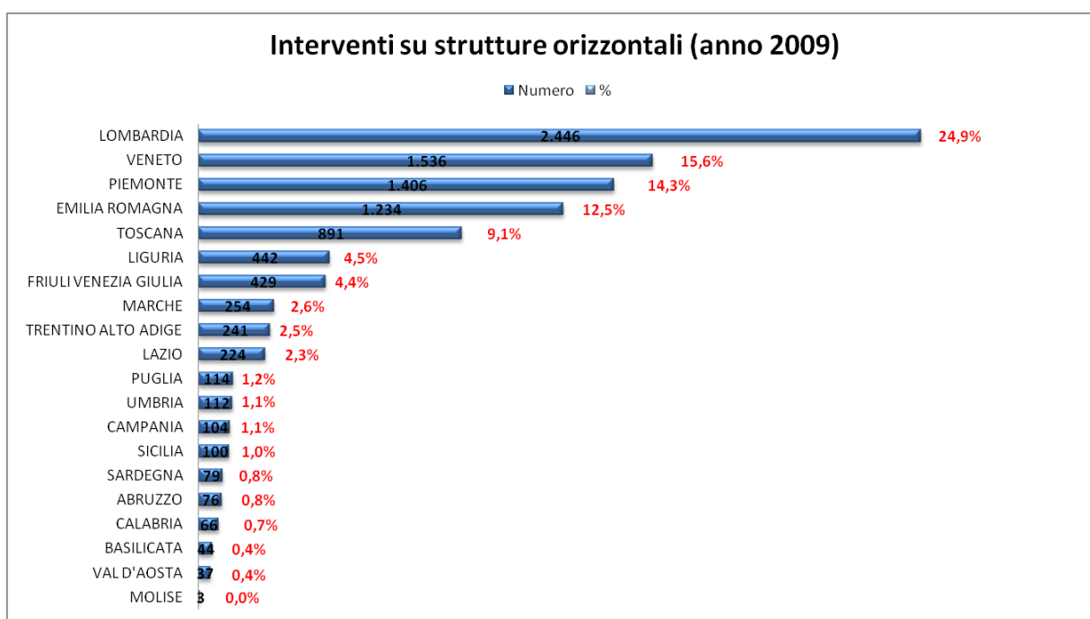
Figura 3.4 Distribuzione per regione degli interventi di coibentazione su strutture opache orizzontali.
