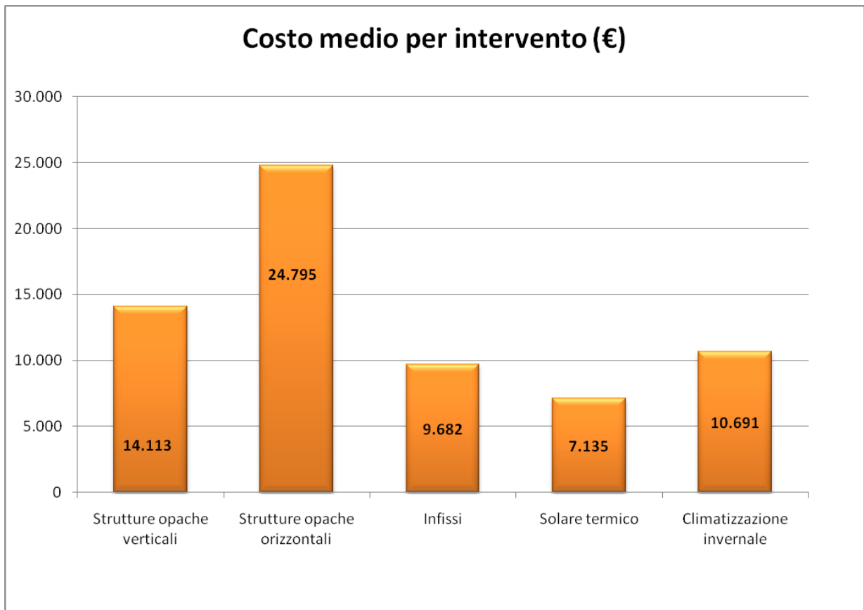
Figura 9: Costo medio di un intervento – Veneto
