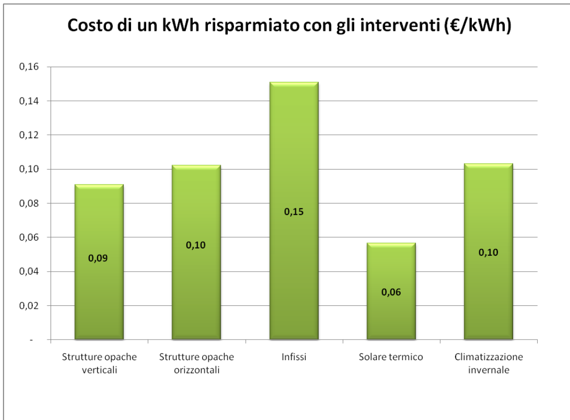
Figura 11: Costo di un MWh annuo risparmiato per tipologia di intervento – Emilia Romagna
