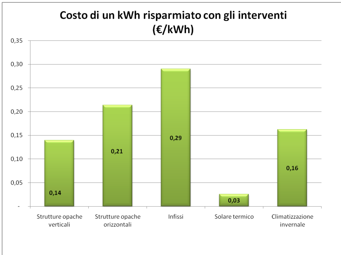
Figura 11: Costo di un MWh annuo risparmiato per tipologia di intervento – Puglia
