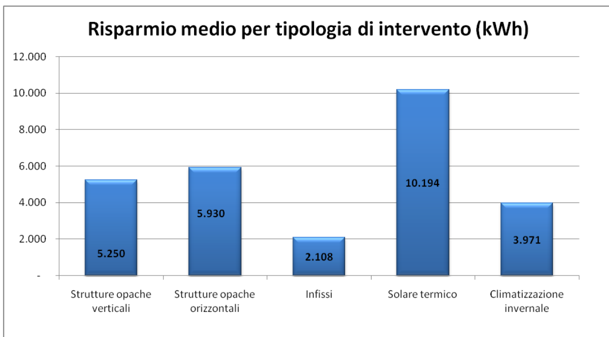
Figura 10: Risparmio medio annuo ottenuto per tipologia di intervento – Calabria
