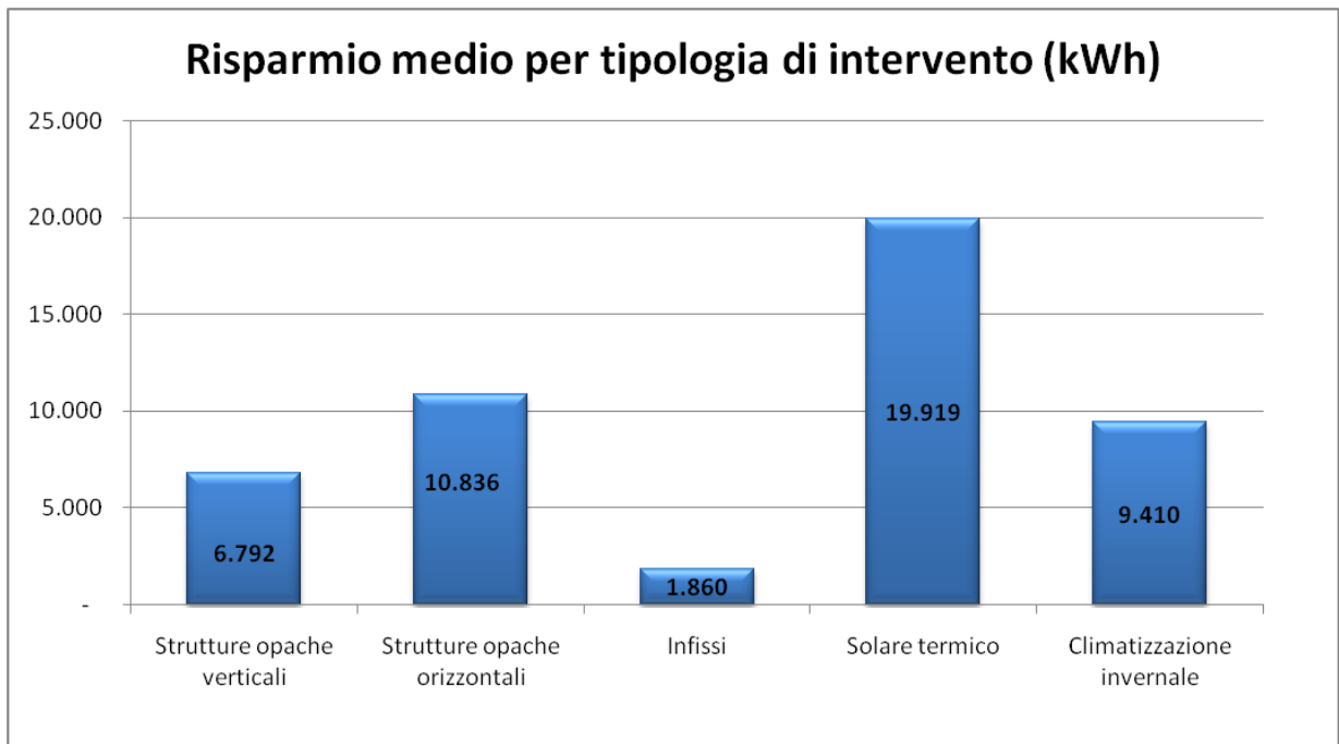
Figura 10: Risparmio medio annuo ottenuto per tipologia di intervento – Toscana
