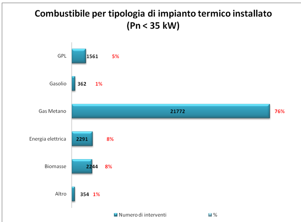
Figura 13: Distribuzione delle pratiche pervenute per tipologia di impianto termico sostituito – Italia I valori numerici sono riferiti alle pratiche inviate prima del 15-08-2009.
