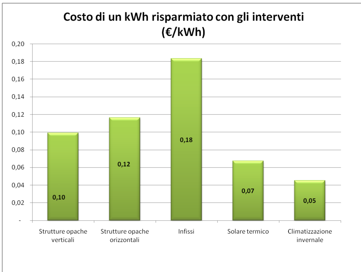
Figura 11: Costo di un MWh annuo risparmiato per tipologia di intervento – Bolzano
