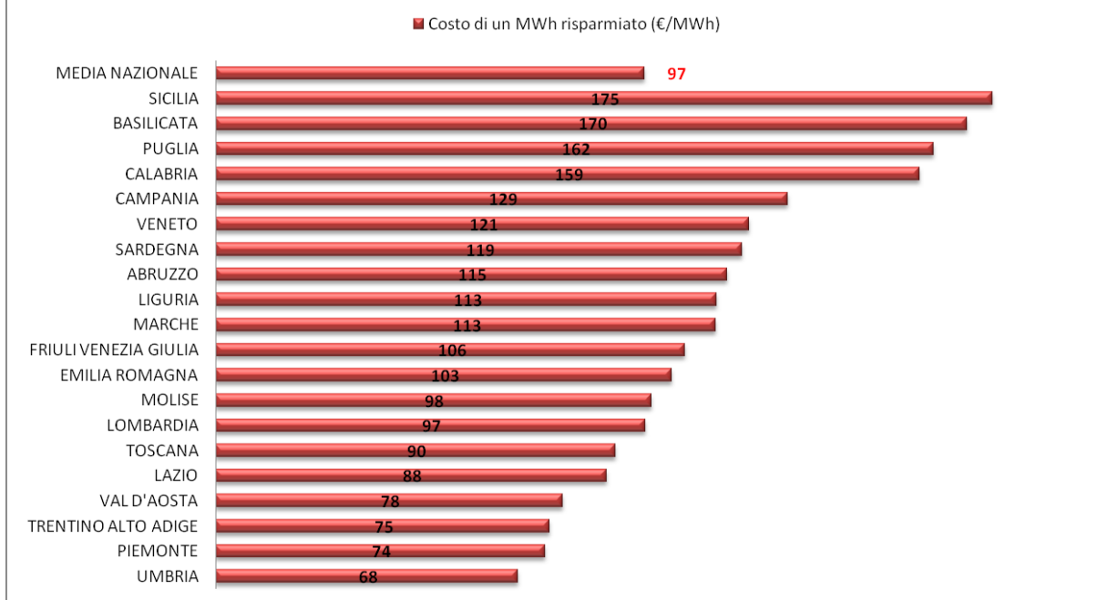
Figura 3.35 Sostituzione di impianti termici. Costo medio di ogni MWh risparmiato con gli interventi. I valori numerici sono riferiti al valore complessivo di pratiche inviate nel 2009.
