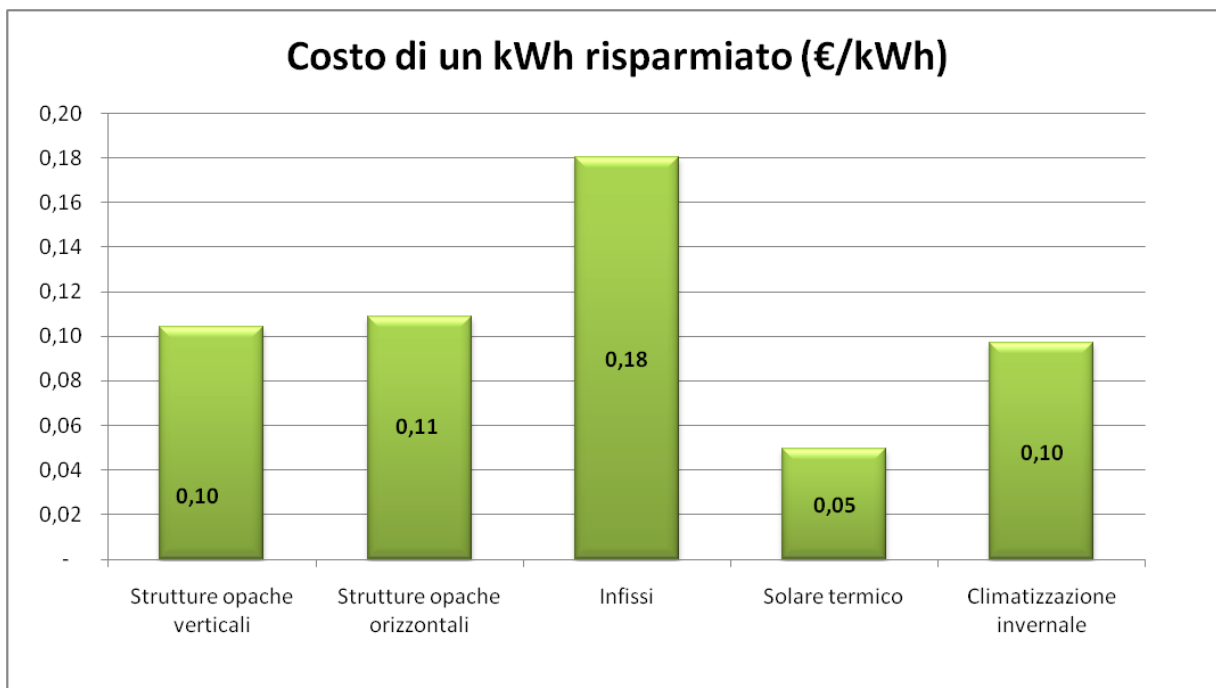
Figura 11: Costo di un MWh annuo risparmiato per tipologia di intervento – Italia
