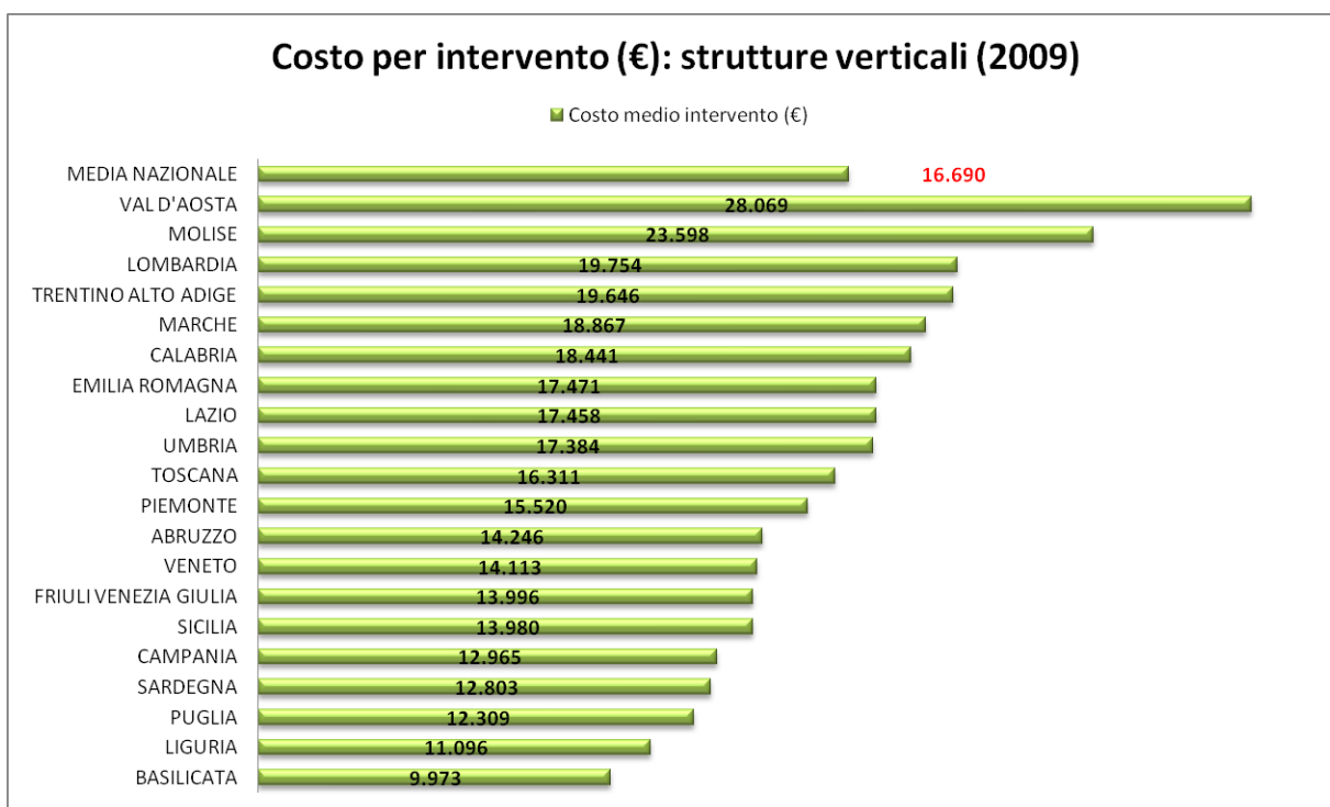
Figura 3.10 Distribuzione regionale del costo medio dell'intervento su strutture opache verticali.
