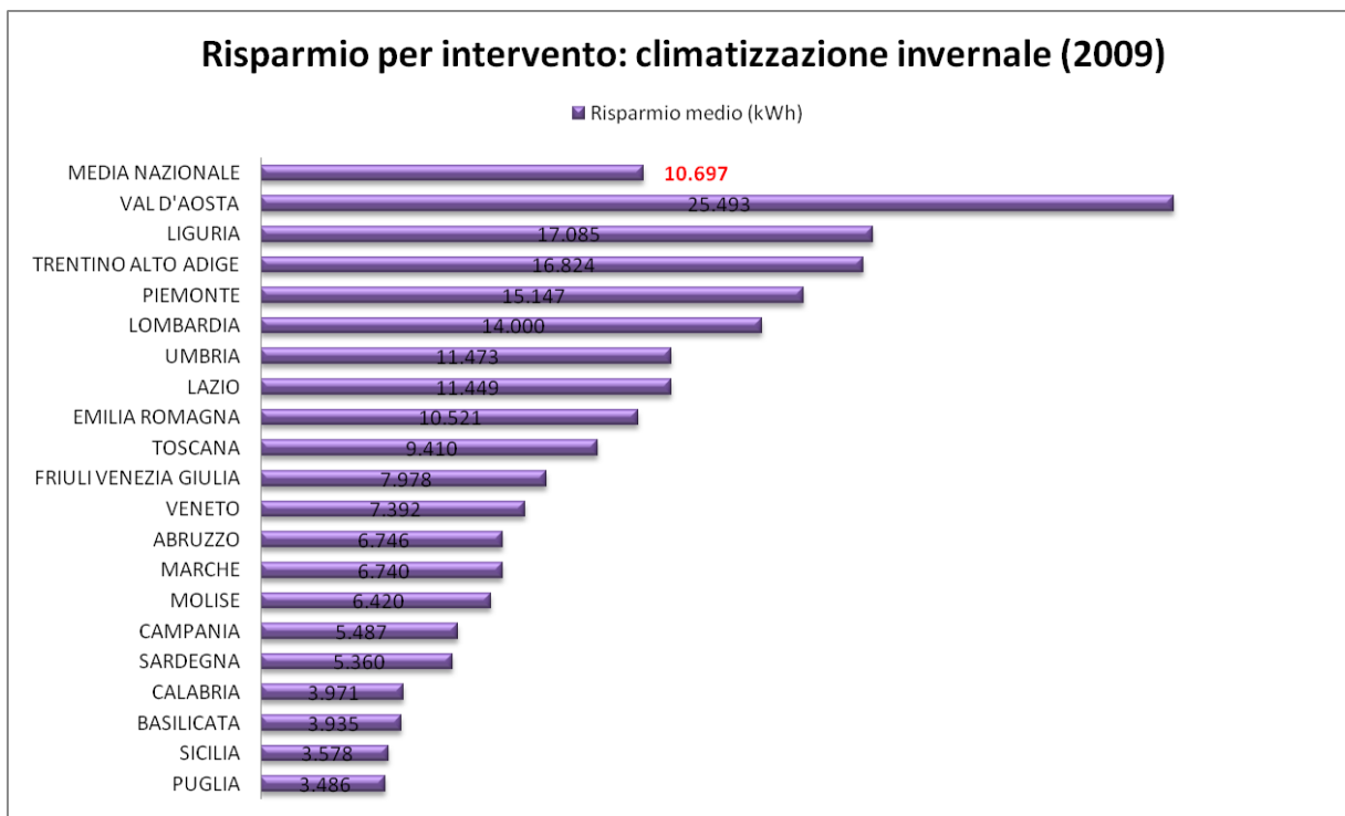
Figura 3.33 Sostituzione di impianti termici. Risparmio realizzato con l'intervento medio. I valori numerici sono riferiti al valore complessivo di pratiche inviate nel 2009.
