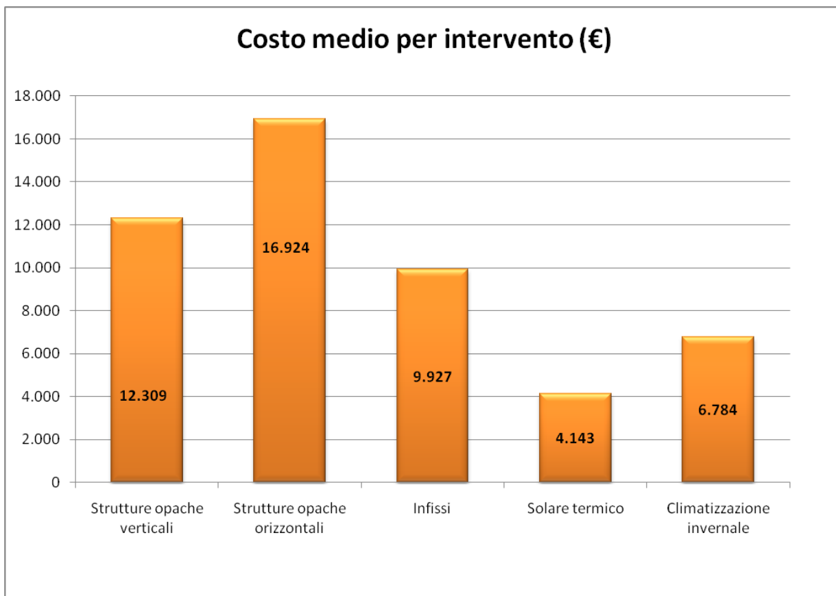
Figura 9: Costo medio di un intervento – Puglia
