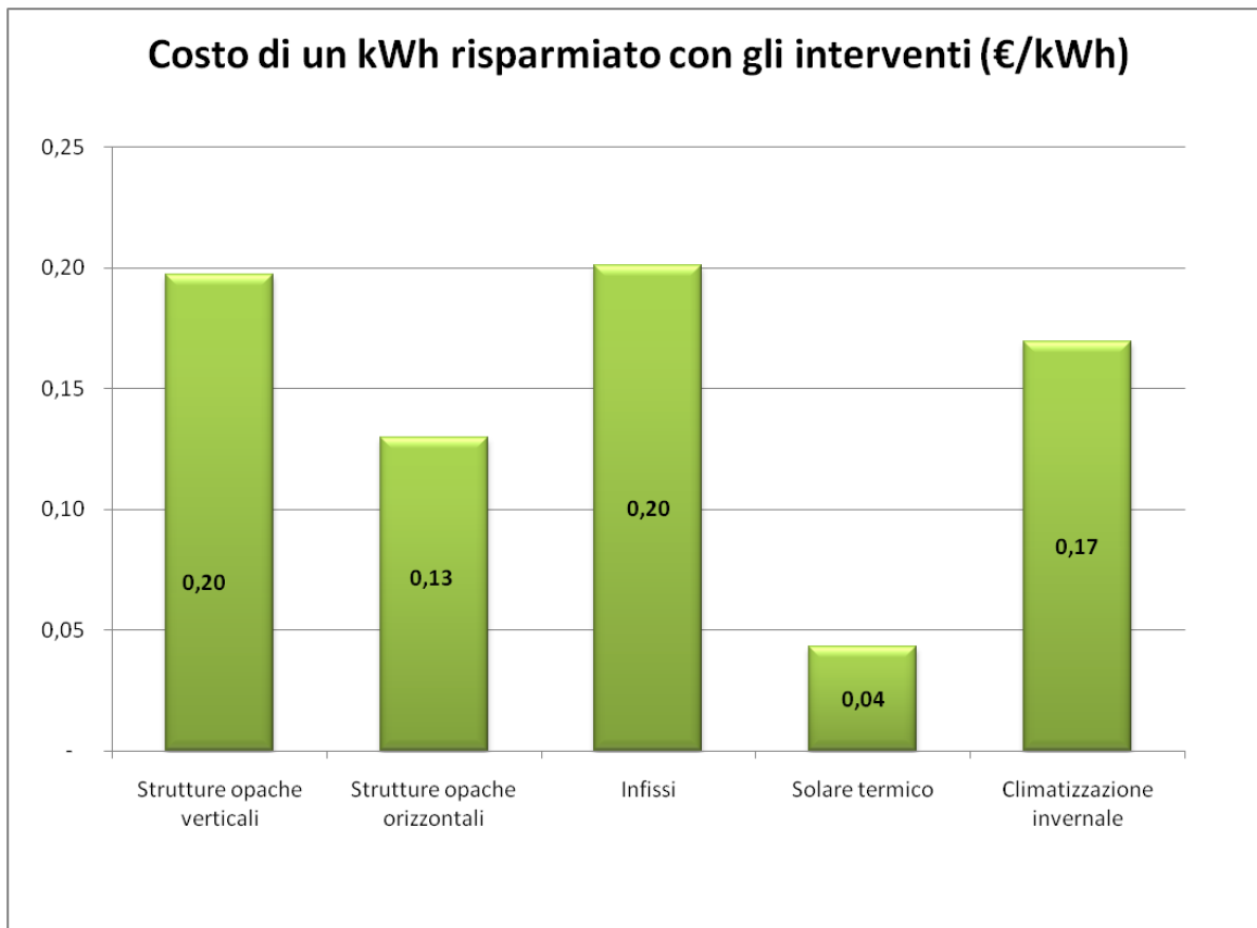
Figura 11: Costo di un MWh annuo risparmiato per tipologia di intervento – Basilicata
