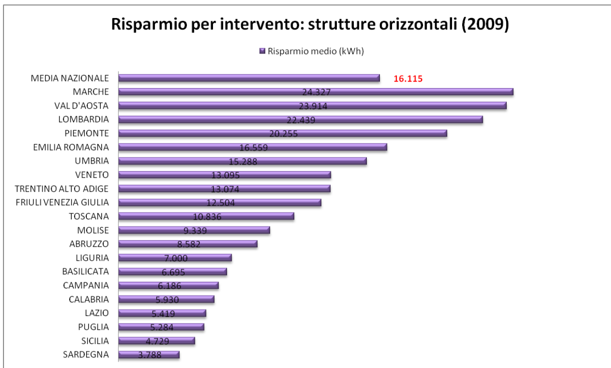
Figura 3.5 Distribuzione per regione del risparmio medio annuo a seguito di interventi su strutture opache orizzontali.
