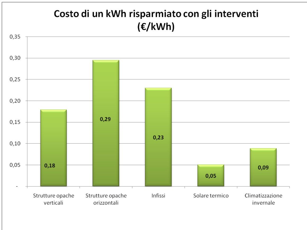
Figura 11: Costo di un MWh annuo risparmiato per tipologia di intervento – Lazio
