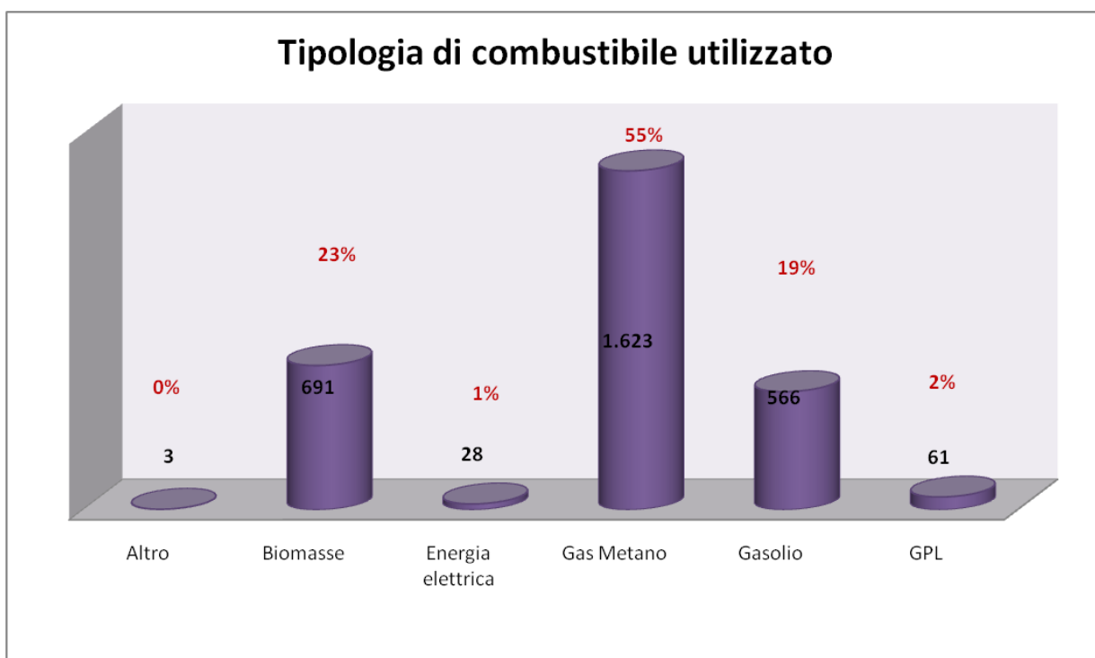
Figura 6: Distribuzione delle pratiche pervenute per tipologia di combustibile utilizzato – Bolzano
