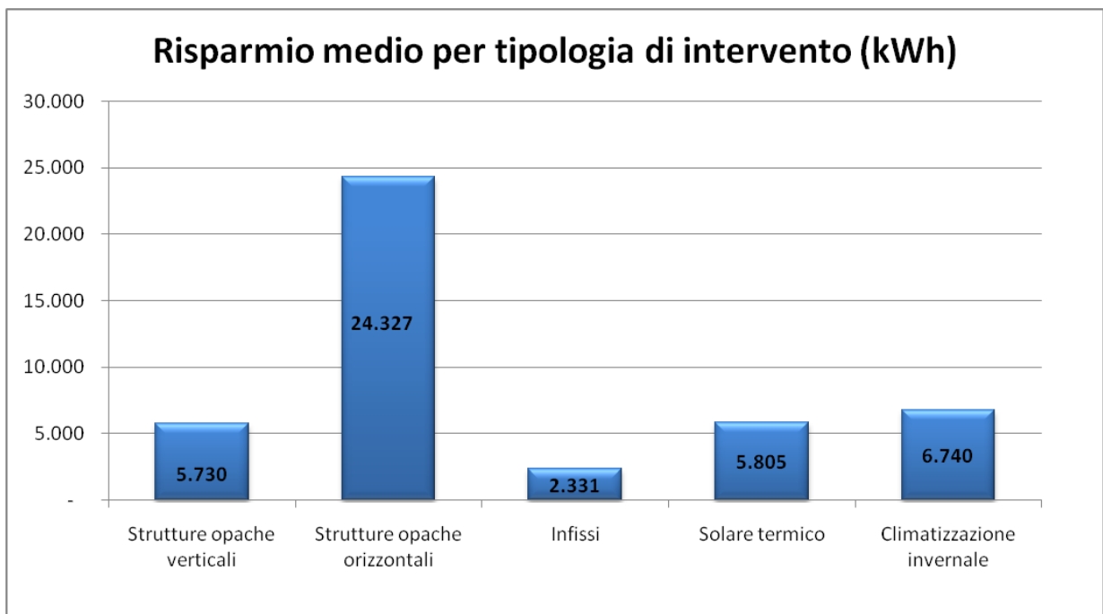
Figura 10: Risparmio medio annuo ottenuto per tipologia di intervento – Marche
