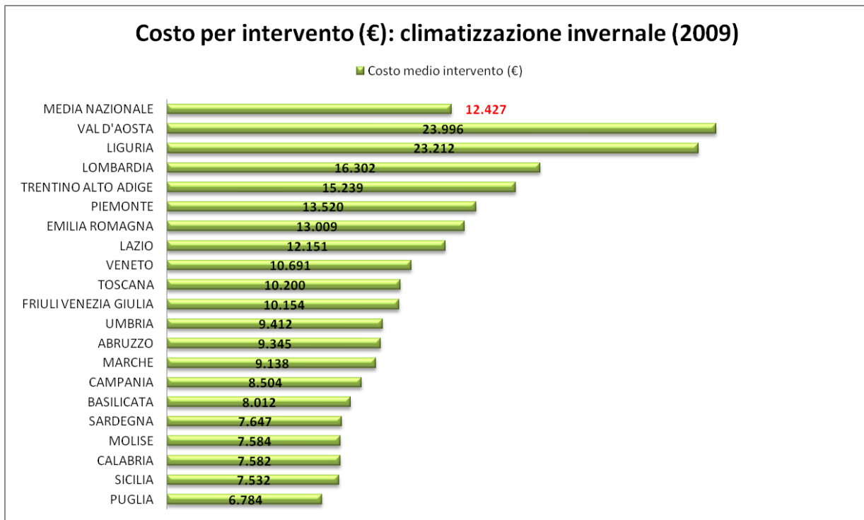
Figura 3.34 Sostituzione di impianti termici. Costo medio dell'intervento. I valori numerici sono riferiti al valore complessivo di pratiche inviate nel 2009.
