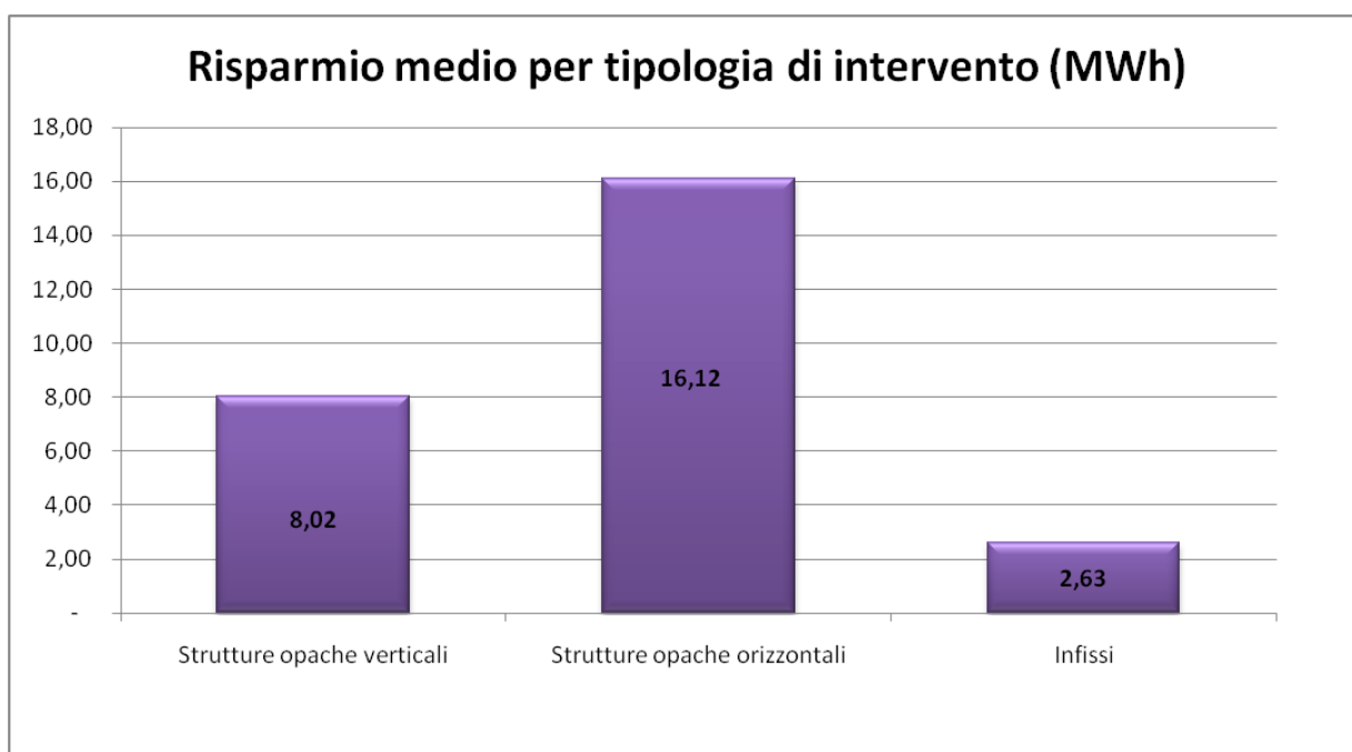
Figura 3.20 Risparmio medio per tipologia di intervento.
