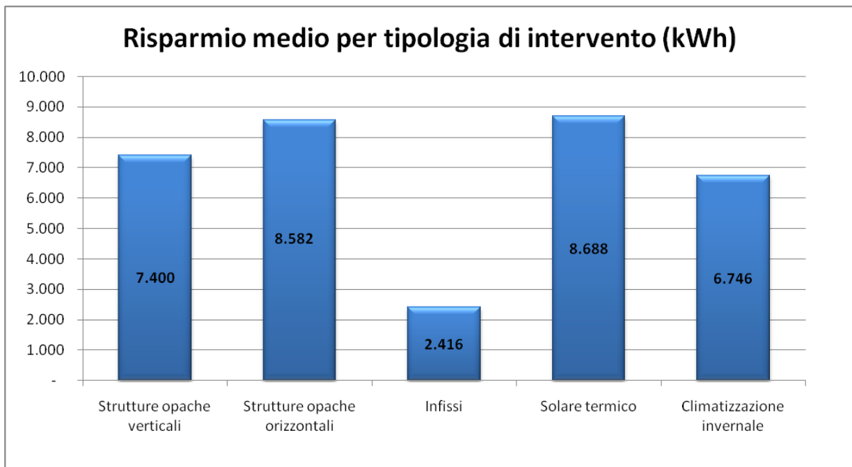
Figura 10: Risparmio medio annuo ottenuto per tipologia di intervento – Abruzzo
