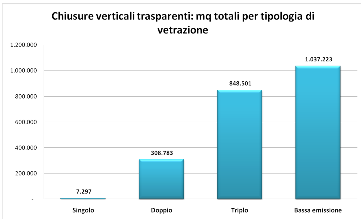
Figura 3.19 Metri quadri totali installati per tipologia di vetrazione.
