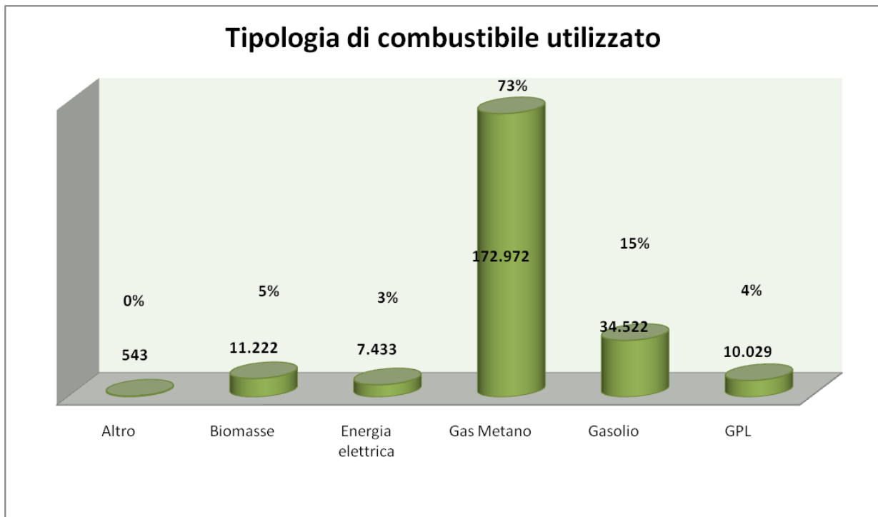
FIG. 2.7 DISTRIBUZIONE DEGLI IMPIANTI TERMICI PER TIPOLOGIA DI COMBUSTIBILE
