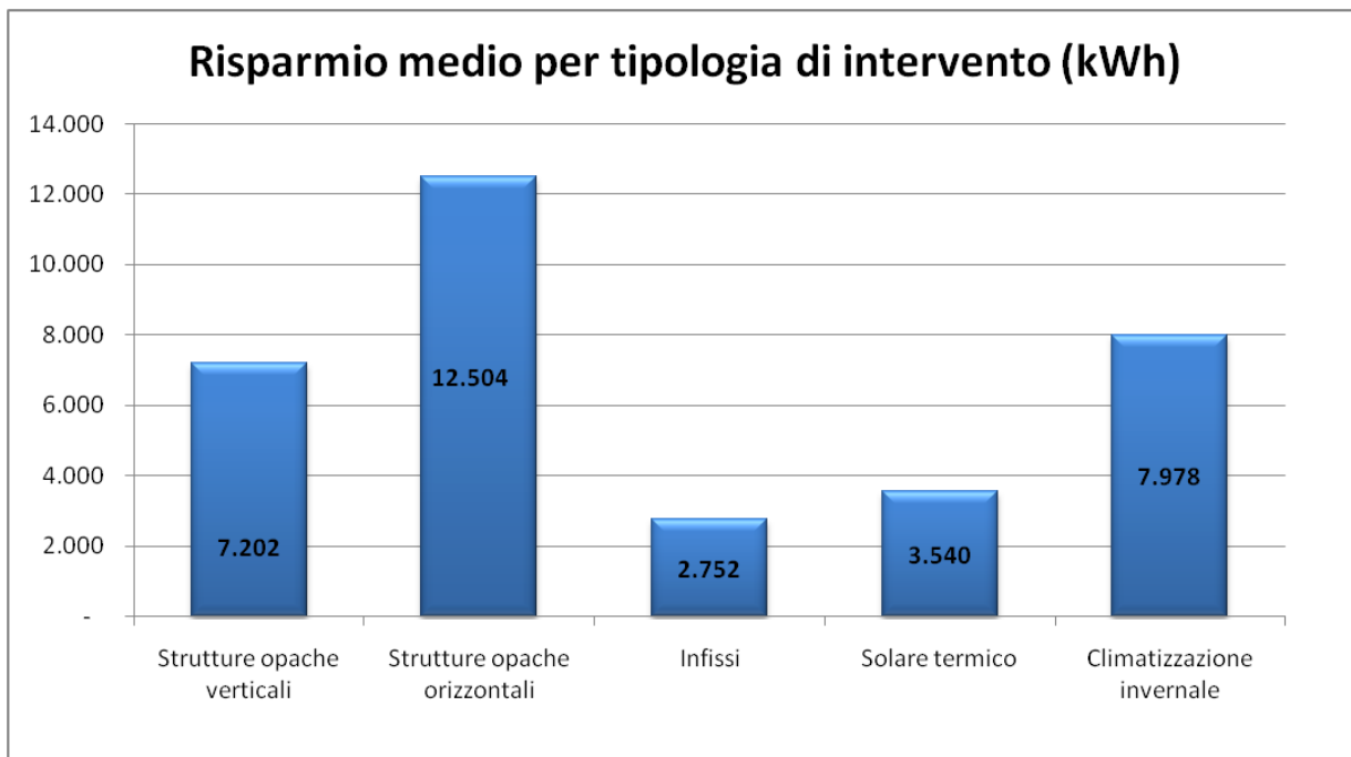
Figura 10: Risparmio medio annuo ottenuto per tipologia di intervento – Friuli VG
