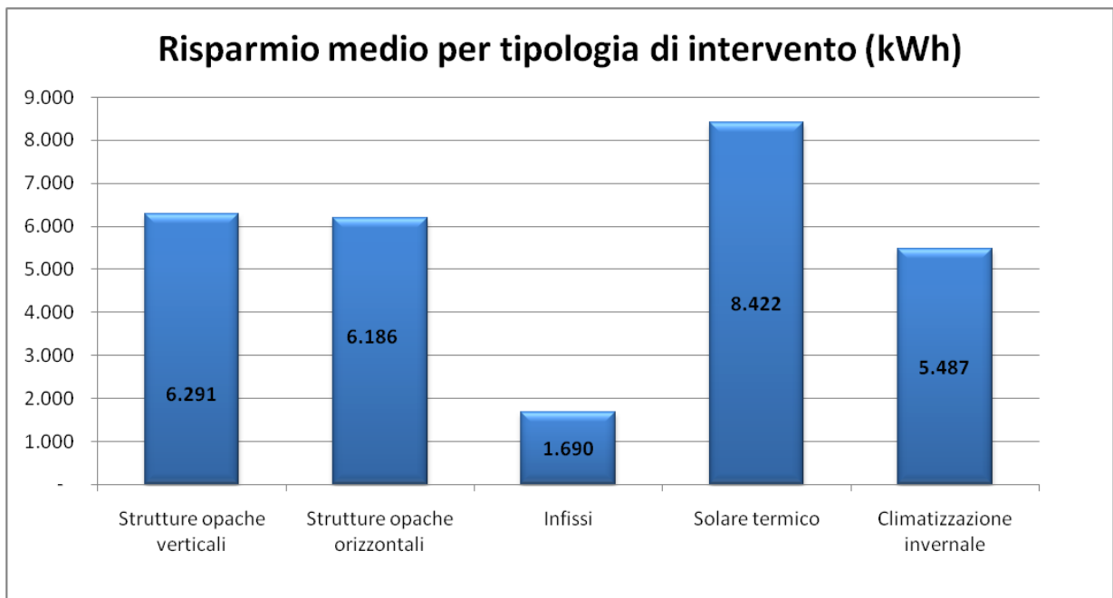
Figura 10: Risparmio medio annuo ottenuto per tipologia di intervento – Campania
