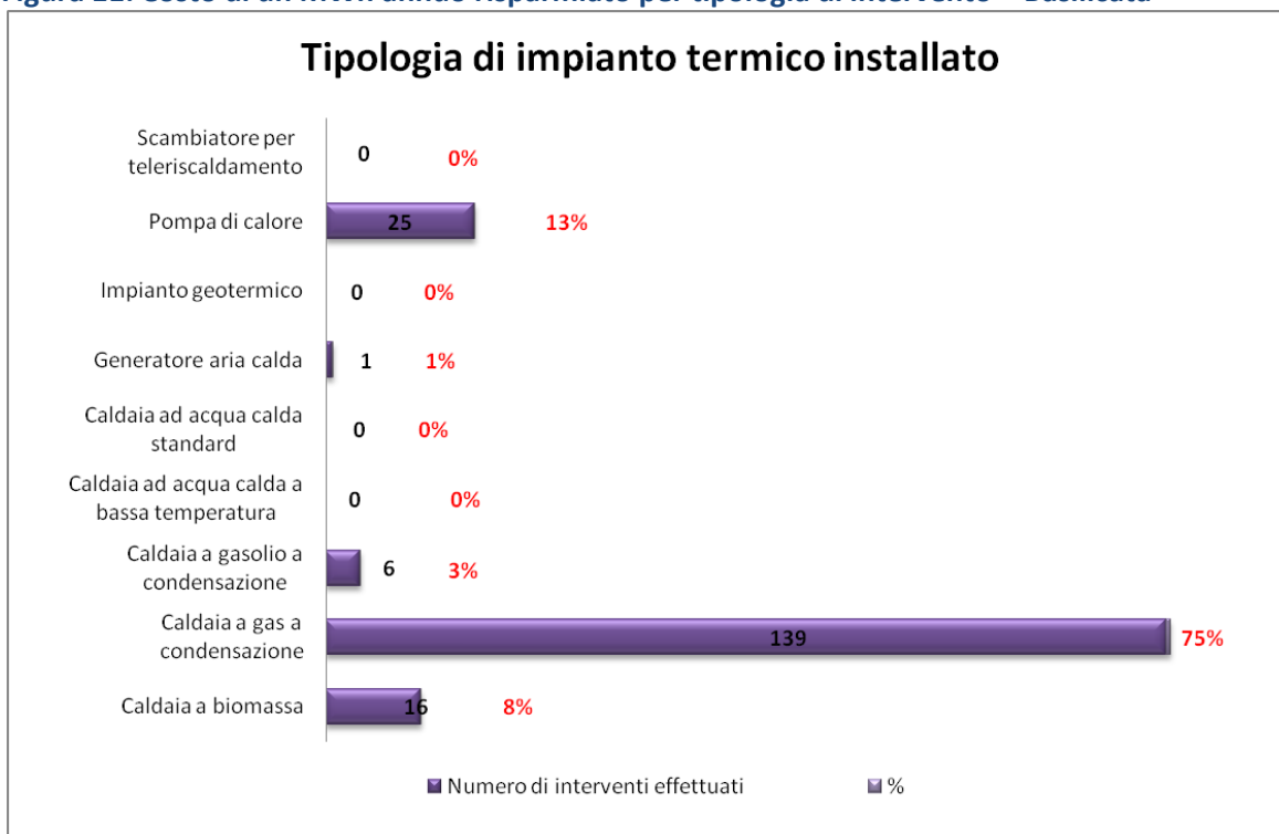
Figura 12: Distribuzione delle pratiche pervenute per tipologia di impianto termico sostituito – Basilicata I valori numerici sono riferiti alle pratiche inviate prima del 15-08-2009.
