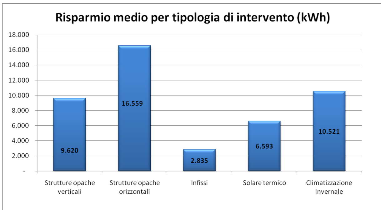
Figura 10: Risparmio medio annuo ottenuto per tipologia di intervento – Emilia Romagna
