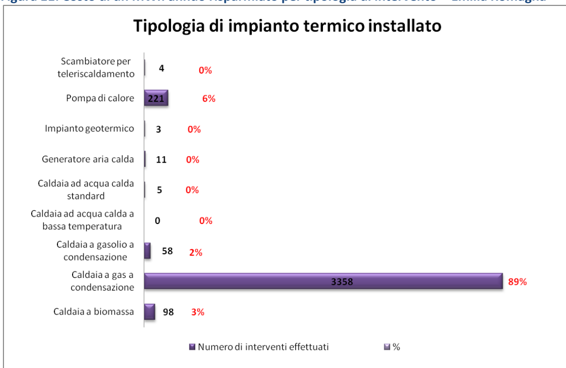
Figura 12: Distribuzione delle pratiche pervenute per tipologia di impianto termico sostituito – Emilia Romagna. I valori numerici sono riferiti alle pratiche inviate prima del 15-08-2009.
