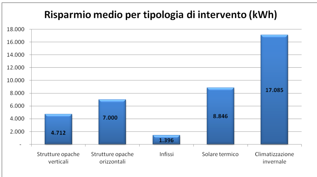
Figura 10: Risparmio medio annuo ottenuto per tipologia di intervento – Liguria
