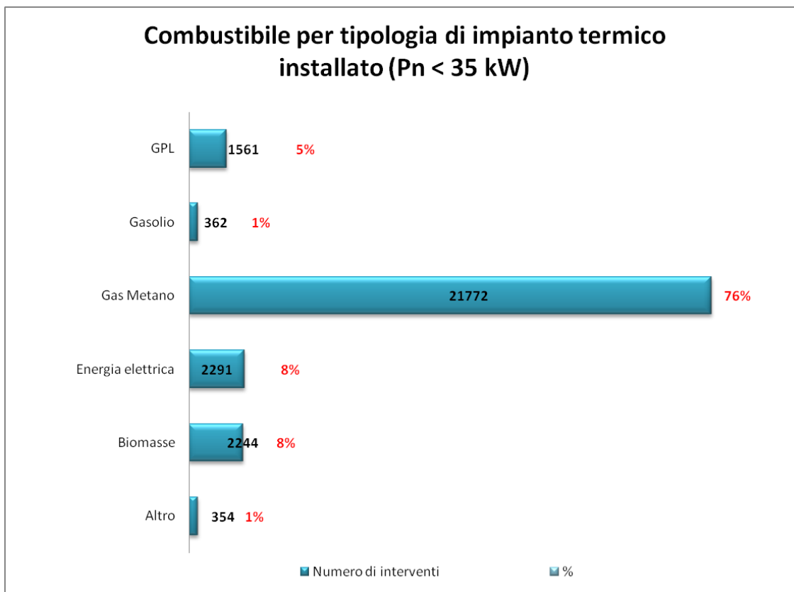
Figura 3.30 Tipologia di combustibile per impianti termici di piccola taglia ( Pn < 35 KW). I valori quantitativi sono riferiti alle pratiche inviate prima del 15-08-2009.
