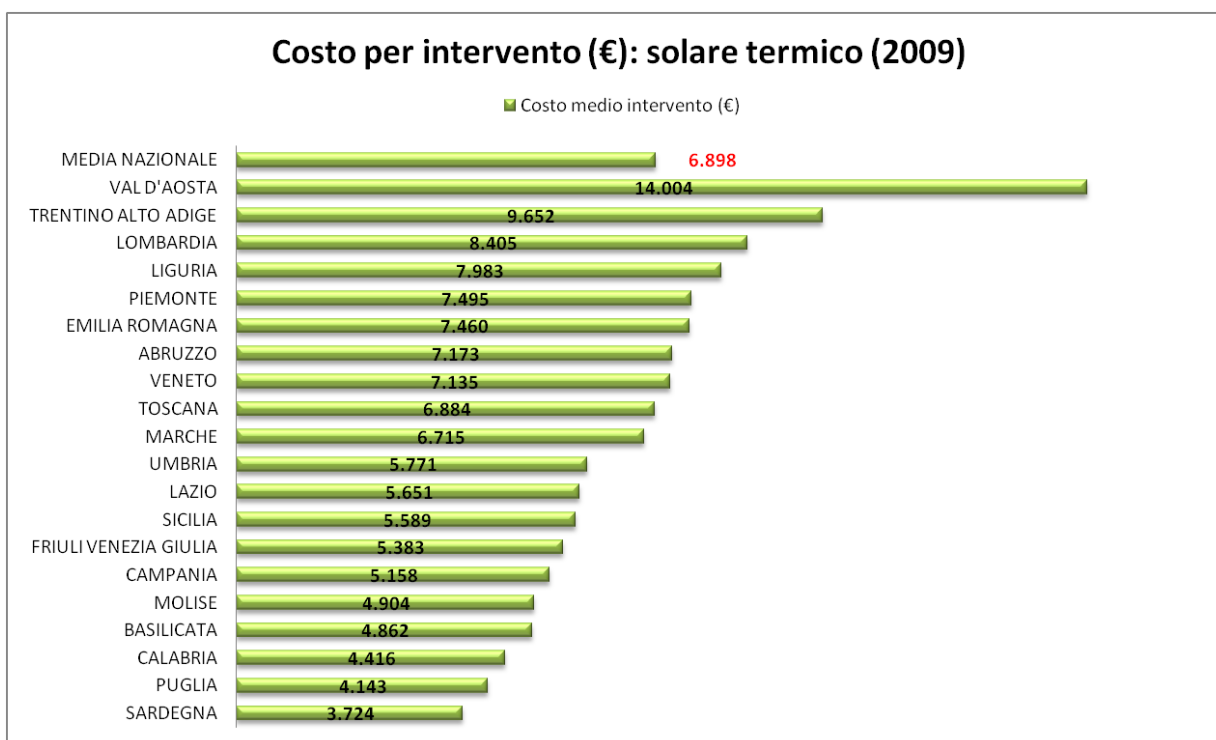
Figura 3.25 Costo medio per l'installazione di un impianto solare termico.
