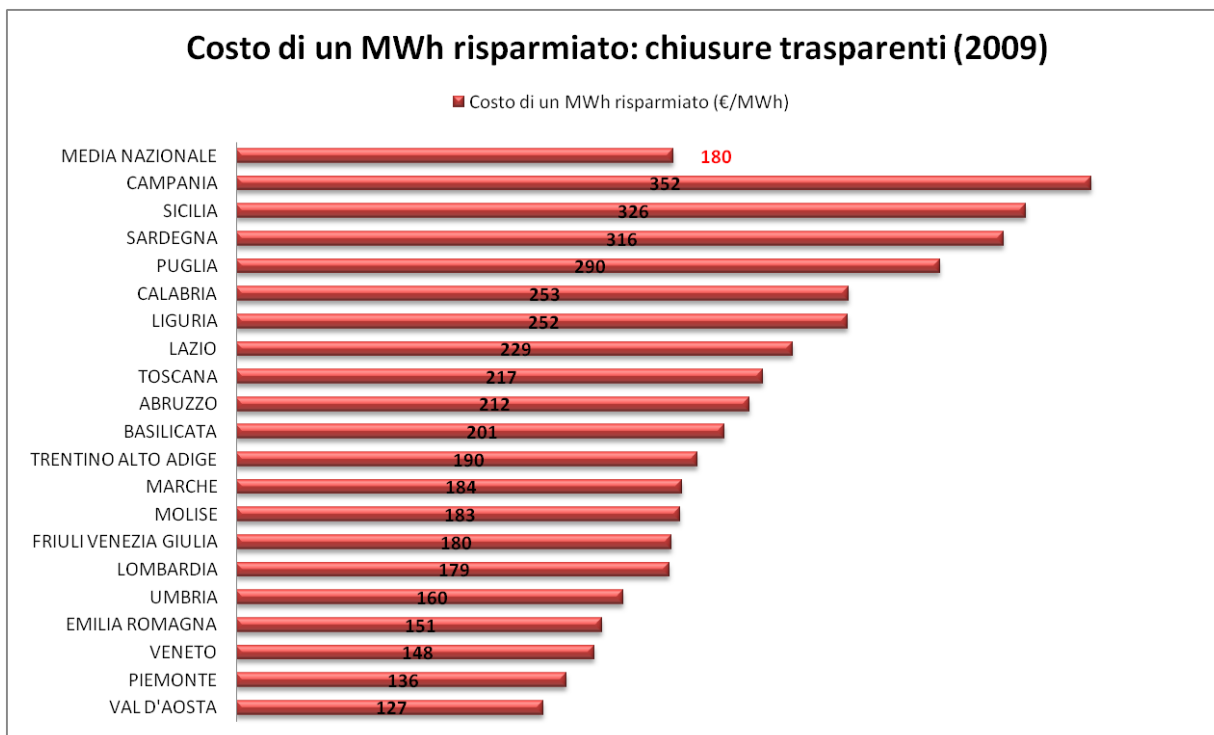
Figura 3.15 Costo medio annuo di ogni MWh risparmiato per la sostituzione di infissi.
