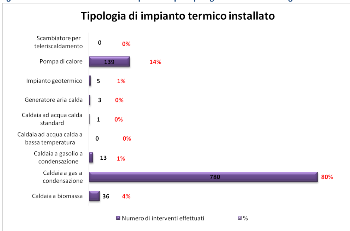
Figura 12: Distribuzione delle pratiche pervenute per tipologia di impianto termico sostituito – Puglia
