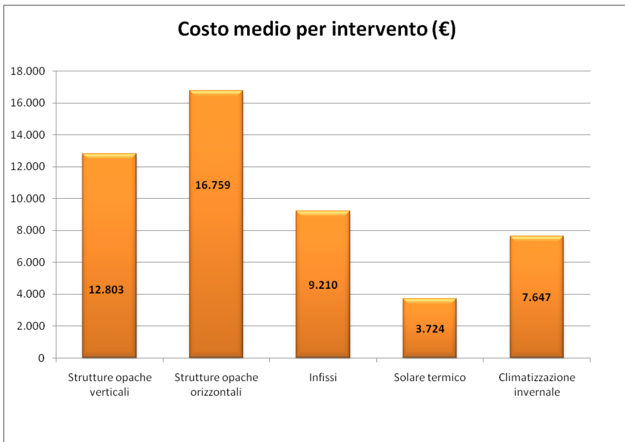
Figura 9: Costo medio di un intervento – Sardegna
