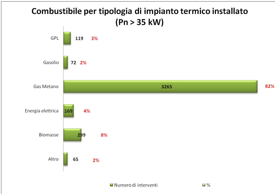
Figura 3.31 Tipologia di combustibile per impianti termici di grande taglia ( Pn > 35 KW). I valori quantitativi sono riferiti alle pratiche inviate prima del 15-08-2009.
