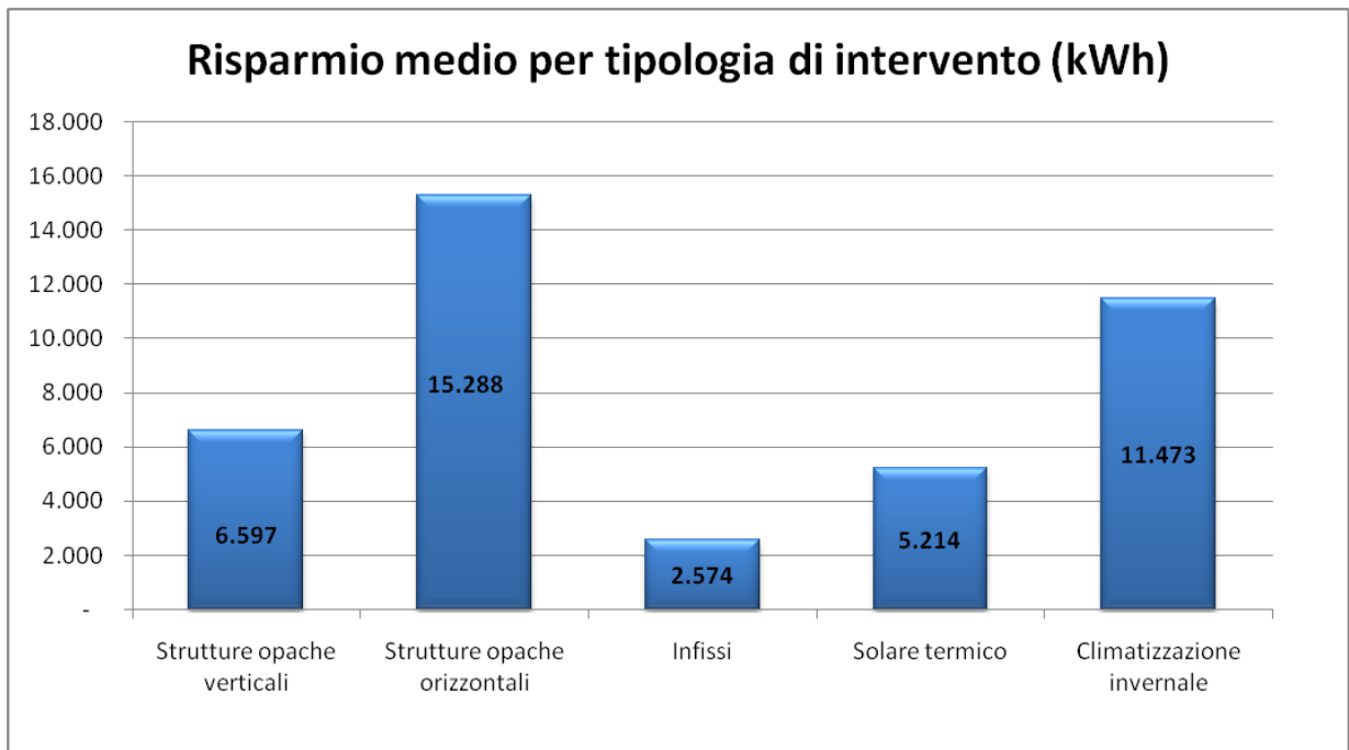
Figura 10: Risparmio medio annuo ottenuto per tipologia di intervento – Umbria
