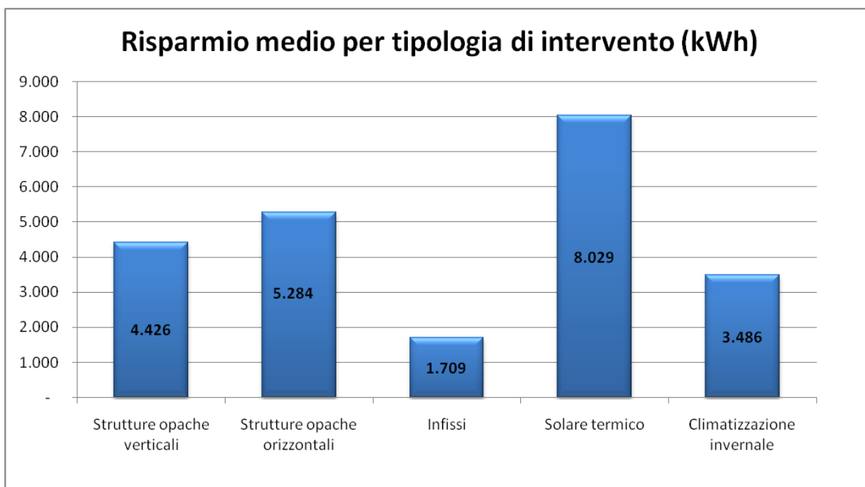
Figura 10: Risparmio medio annuo ottenuto per tipologia di intervento – Puglia
