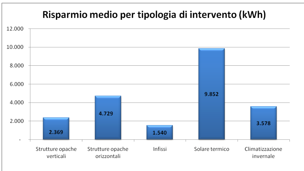
Figura 10: Risparmio medio annuo ottenuto per tipologia di intervento – Sicilia
