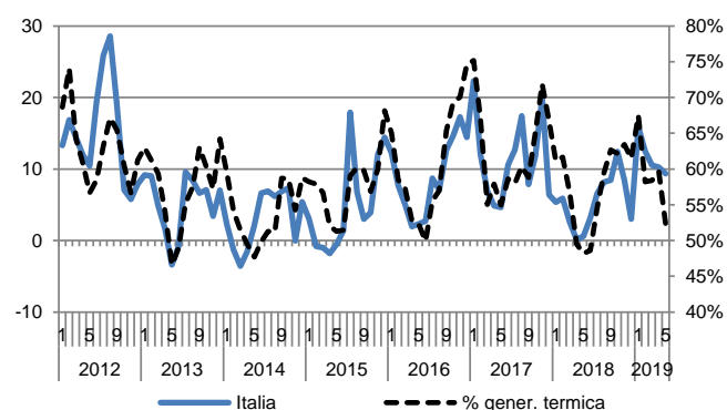
Figura 4.35 - Spark spread 2008-2018 per il sistema Italia (€/MWh, asse sn) e quota di produzione termoelettrica (% , asse dx)
