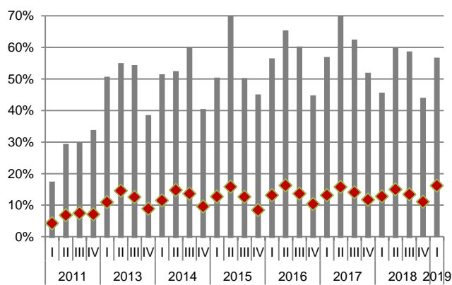
Figura 4.29 - Massima variazione oraria fonti intermittenti (% sul carico e media mobile a 4 termini)
