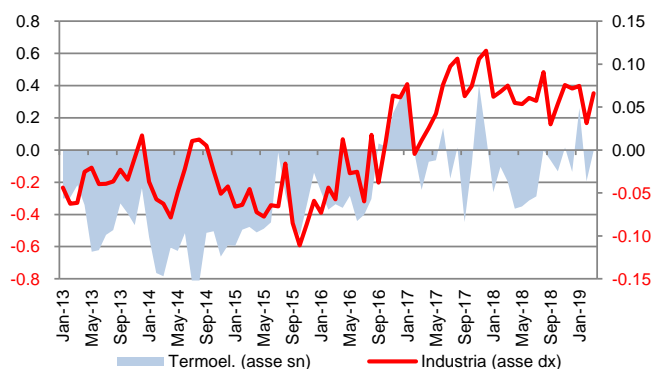
Figura 4.17 - Domanda mensile di gas naturale per settore in Italia – Differenza rispetto alla media decennale (miliardi di m 3 )
