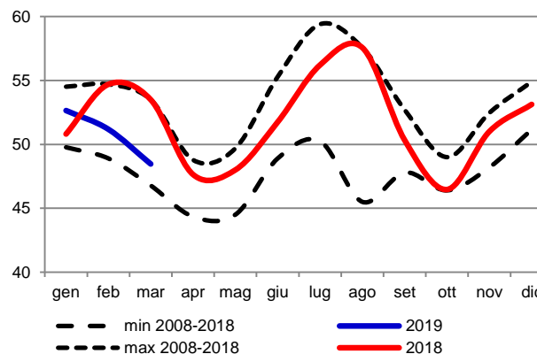
Figura 4.25 - Punta di domanda in potenza (GW)
