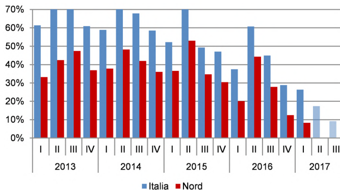
Figura 58 – Capacità di generazione elettrica in eccesso (1% delle ore più critiche)
