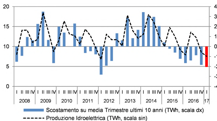
Figura 14 – Produzione idroelettrica (TWh, asse sn) e variazione dai valori medi trimestrali 2006-2016 (TWh, asse dx)
