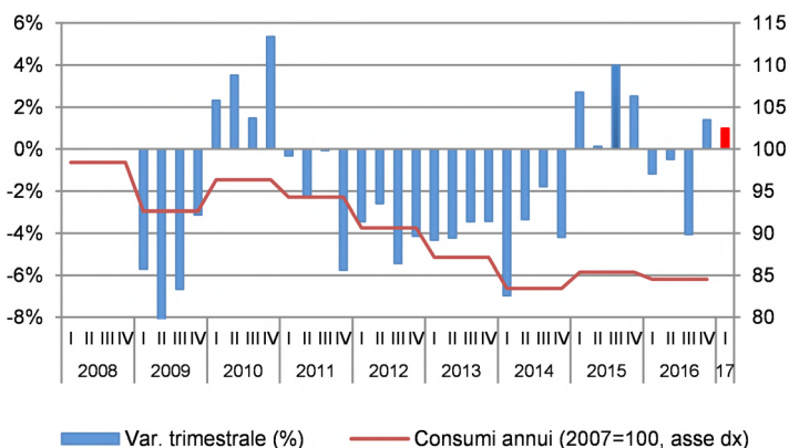
Figura 9 – Consumi di energia primaria trimestrale (var. % su anno prec., asse sn) e annuale (2007=100, asse dx)
