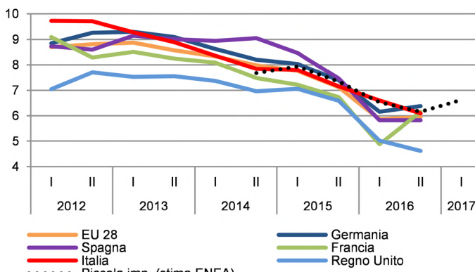
Figura 83 – Prezzo gas per l'industria al netto di tasse e imposte deducibili - consumo annuo 1.000.000-4.000.000 GJ (€/GJ)
