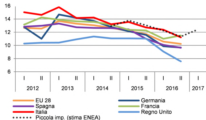
Figura 81 – Prezzo del gas per l'industria al netto di tasse e imposte deducibili: consumo annuo 1.000-10.000 GJ (€/GJ)
