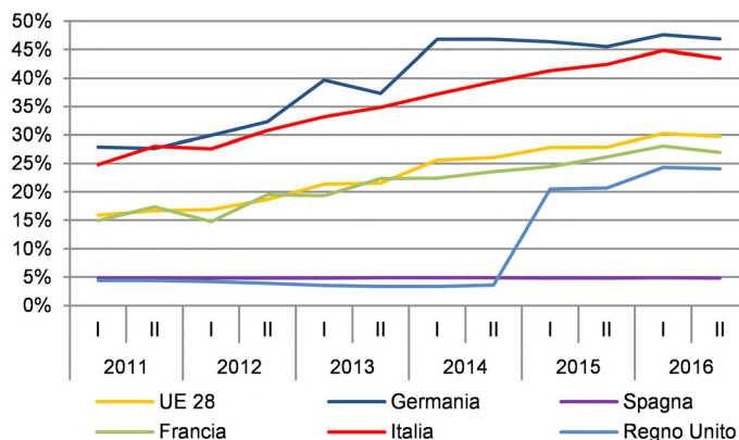
Figura 72 – Percentuale di tasse e imposte non deducibili sul prezzo finale dell'energia (al netto di IVA e imposte deducibili): consumi tra 500-2.000 MWh
