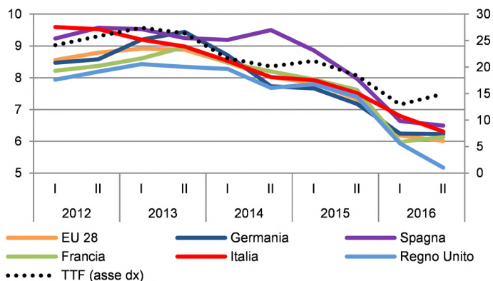
Figura 79 – Prezzo del gas per l'industria al netto di tasse e imposte, consumo annuo 100.000-1.000.000 GJ, e prezzo spot sul TTF (asse sn €/GJ, asse dx €/MWh)
