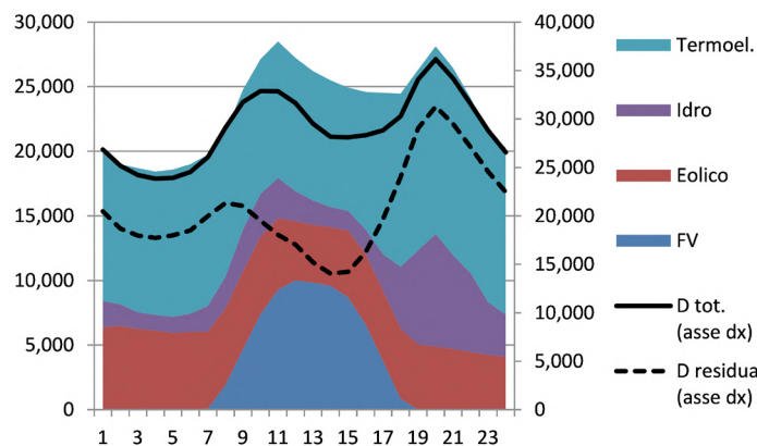
Figura 62 – Diagramma della domanda oraria, della sua copertura e della domanda residua nel giorno di massima penetrazione di FRNP (MW)
