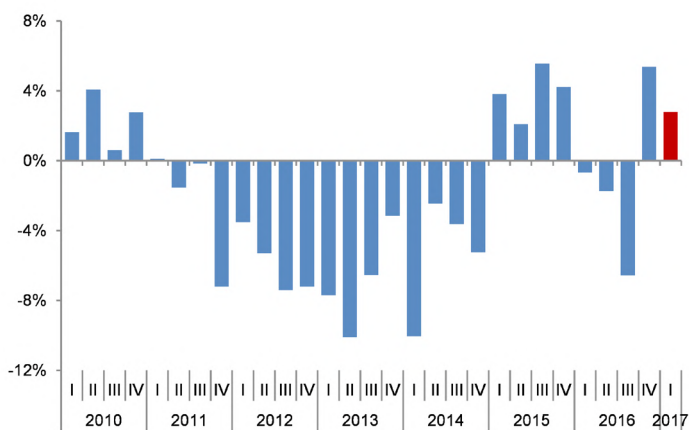
Figura 19 – Emissioni totali di CO 2 del sistema energetico italiano (Variazione tendenziale %)
