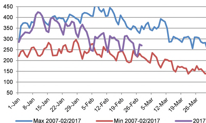
Figura 39 – Domanda giornaliera di gas naturale (MSm 3 )
