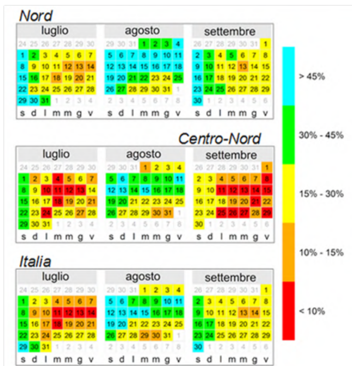
Figura 59 – Minimo orario di capacità di generazione elettrica in eccesso – Simulazione relativa al III trimestre 2017, ipotesi di alta domanda e bassa produzione da FRNP (%)
