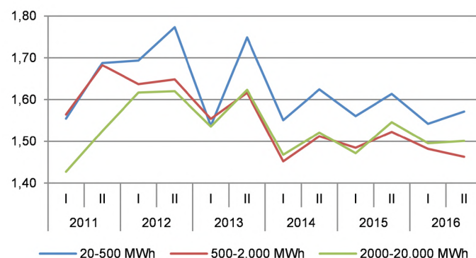
Figura 73 – Percentuale di tasse e imposte non deducibili sul prezzo finale dell'energia elettrica (al netto di IVA e imposte deducibili): scostamento rispetto alla media UE
