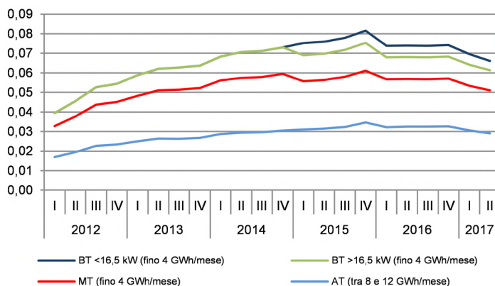
Figura 76 – Oneri di sistema (componenti variabili) consumatori industriali, bassa, media e alta tensione (€/kWh)
