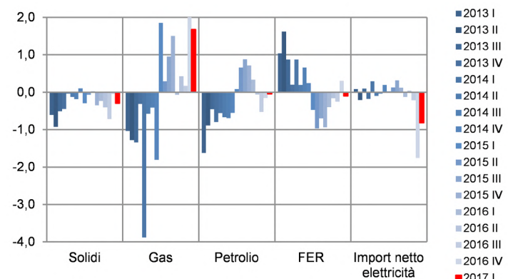
Figura 11 – Fabbisogno energia primaria per fonte (var. trimestre su trimestre anno prec., Mtep)
