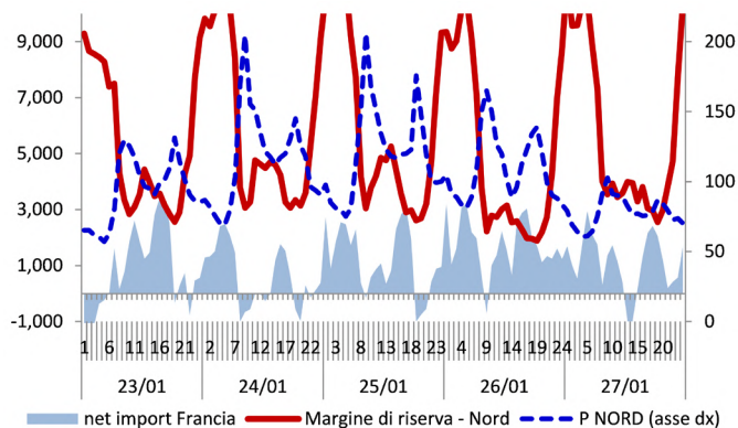
Figura 56 – Import dalla Francia e margine di riserva (MW, asse sn), prezzi orari (€/MWh, asse dx) - zona Nord
