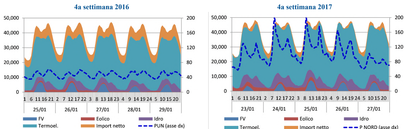
Figura 55 – Diagramma di copertura del fabbisogno orario e prezzi sulla borsa elettrica - Gennaio 2016 e Gennaio 2017
