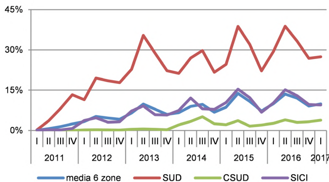
Figura 63 – Indice ENTSO-E sulla flessibilità del sistema: % delle ore in cui la variazione oraria della produzione intermittente > 10% della domanda
