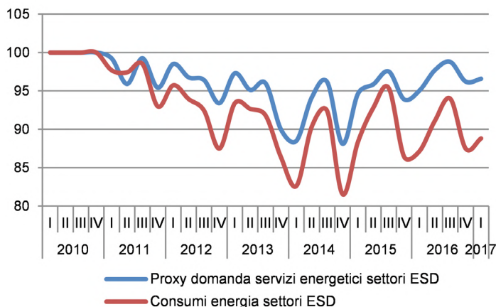
Figura 24 – Consumi energia e proxy domanda di servizi energetici dei settori ESD
