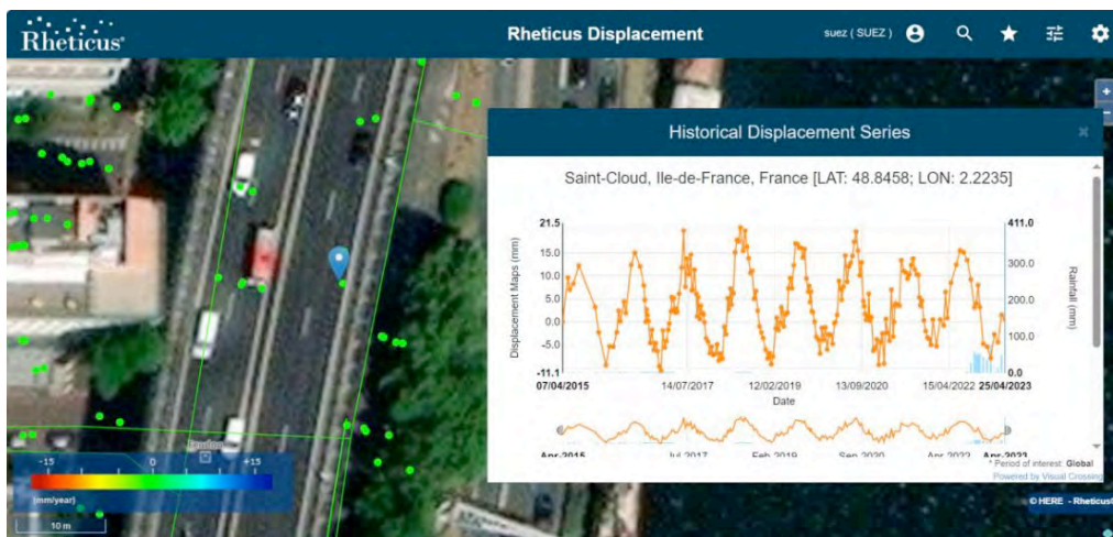
FIGURA 4 - Andamento stagionale dei movimenti analizzati nel portale Rheticus® Displacement
