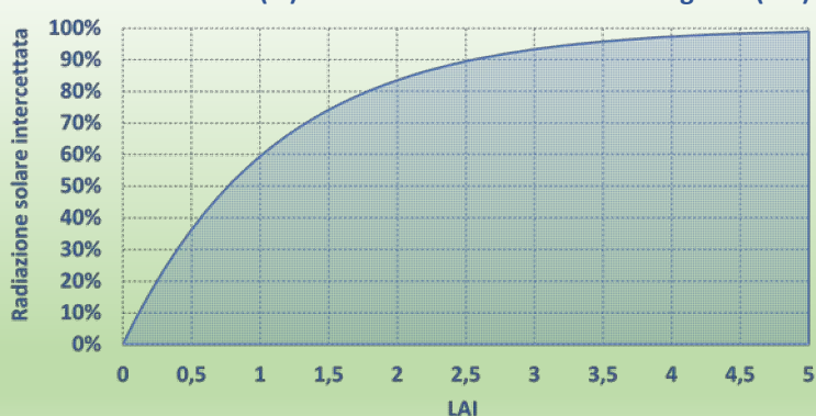
Figura 5.3 – Radiazione solare intercettata (%) al variare dell'Indice di Area Fogliare (LAI)
