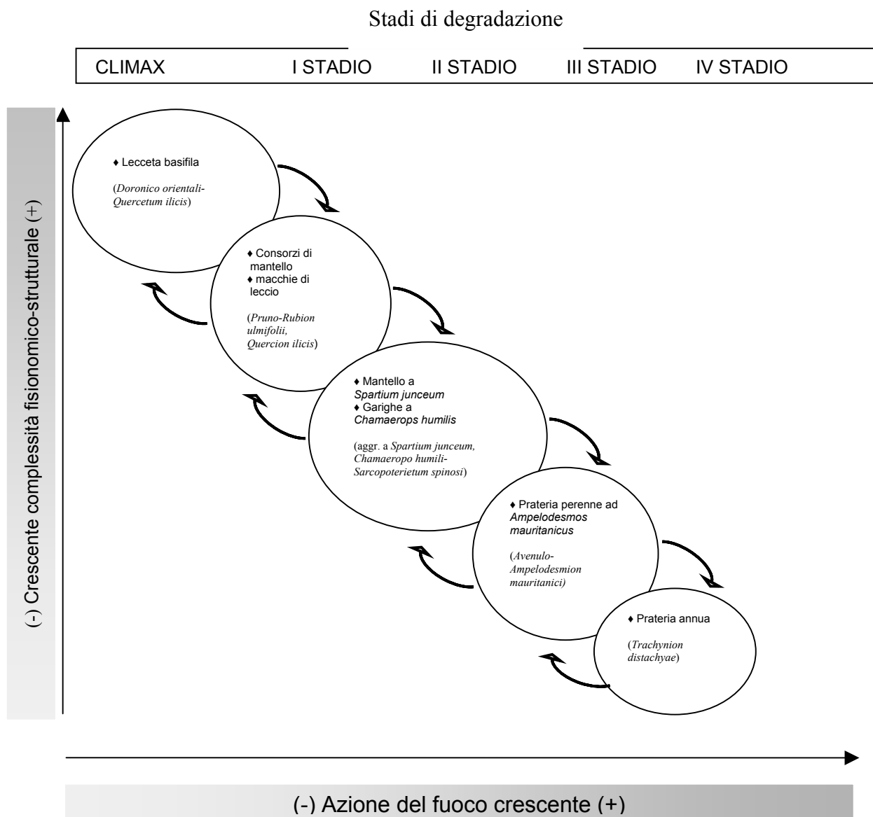
Figura 16 - Schema della dinamica della vegetazione basifila del piano mesomediterraneo dei Monti Iblei (Sicilia); tra parentesi vengono riportate le corrispondenti unità fitosociologiche
