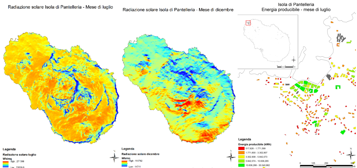
Figura 12.6 a) Irradiazione solare media mensile per l'isola di Pantelleria calcolata nei mesi di luglio e dicembre (Wh/m 2 ); b) energia elettrica producibile nel mese di luglio (kWh)
