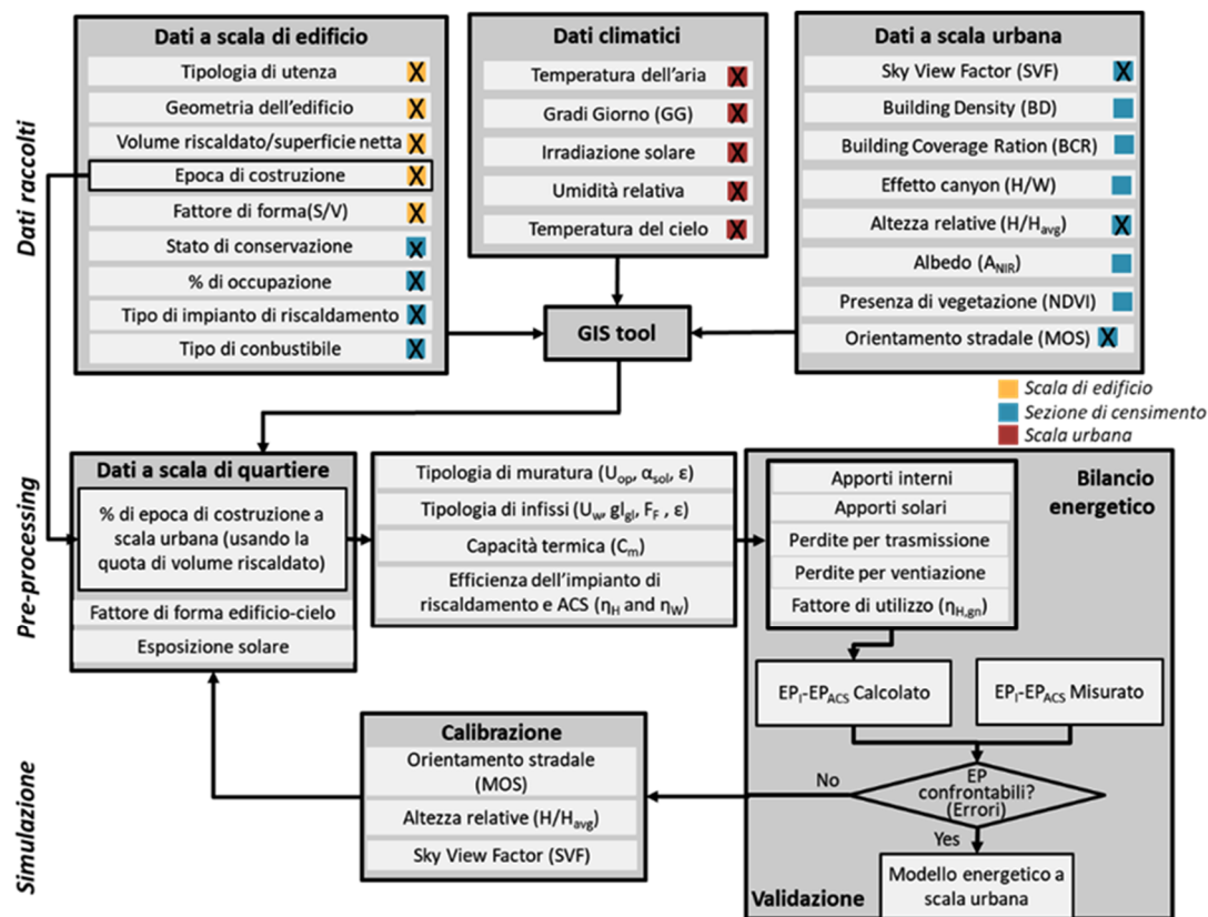
Figura 3.3 Metodologia di calcolo: dati di input (a scala di edificio e a scala urbana & dati climatici), pre-processing (a scala di distretto), simulazione e validazione del modello di consumo per edifici residenziali
