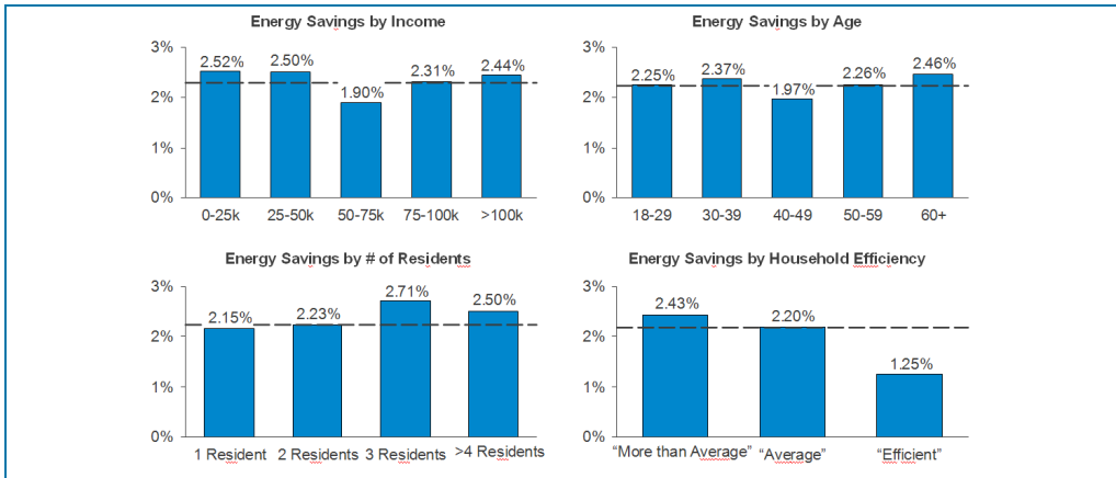
Figura 18 – Risparmi energetici ottenuti con programmi di efficienza comportamentale, per tipologia di utente
