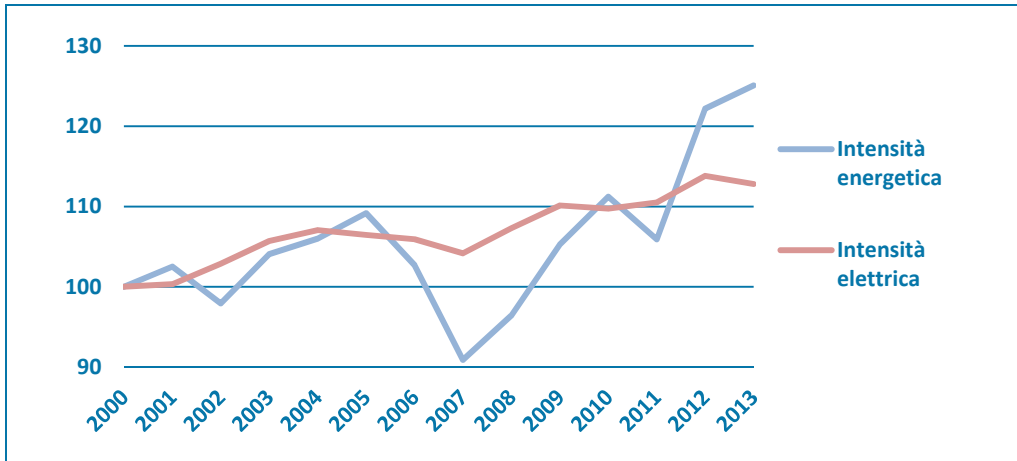
Figura 11 – Intensità energetica ed elettrica nel residenziale (2000=100), anni 2000-2013
