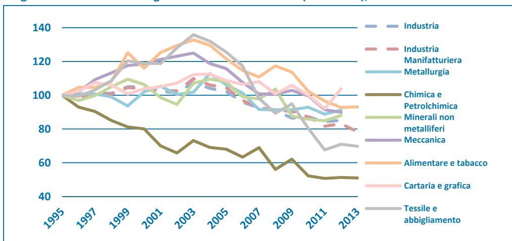
Figura 10 – Intensità energetica finale nell’industria (1995=100), anni 1995-2013
