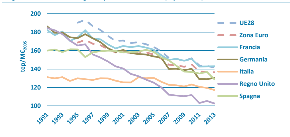
Figura 9 – Intensità energetica primaria nell’UE28 (tep/M€ 2005 ), anni 1991-2013
