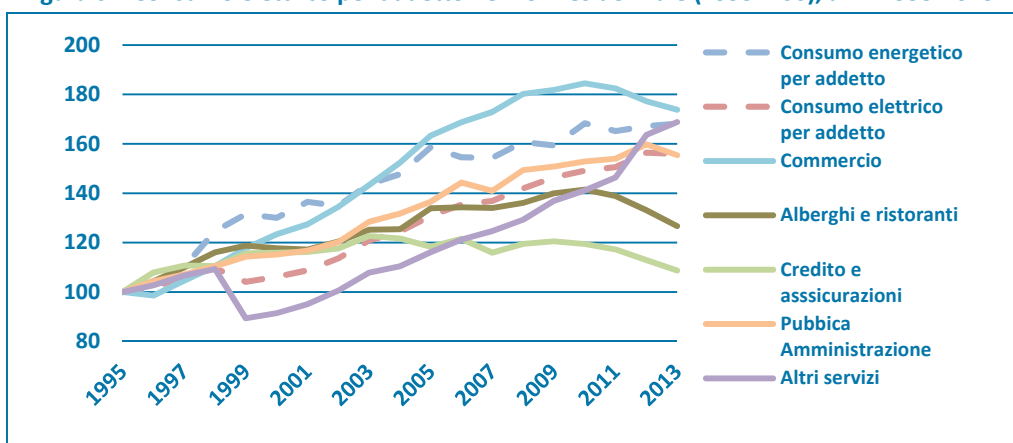
Figura 6 – Consumo elettrico per addetto nel non residenziale (1995=100), anni 1995-2013
