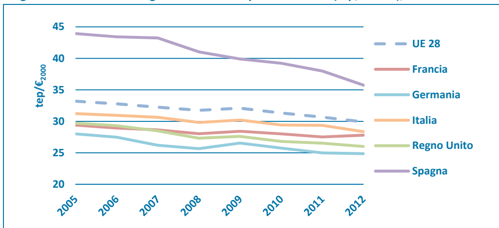
Figura 13 – Intensità energetica settore trasporti nell'UE28 (tep/M€ 2000 ), anni 2005-2012
