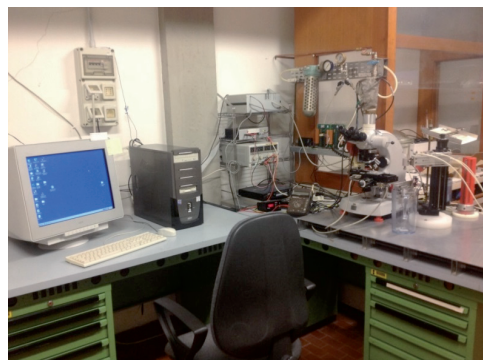
Sistema di misura del Servizio Radon ENEA
